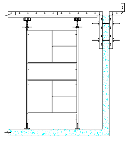
3ª ETAPA LAJE COM BEIRAL
