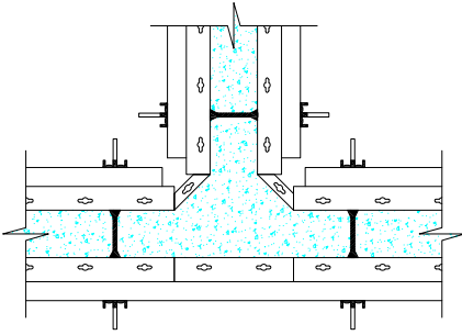
PAREDE EM 'T' COM MÍSULA
